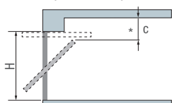
BC – Brama uchylna wysunięta, częściowo cofnięta
