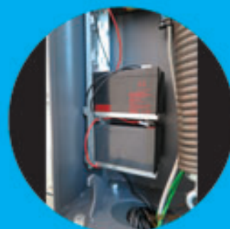
Pomocniczy system zasilania na akumulatory
